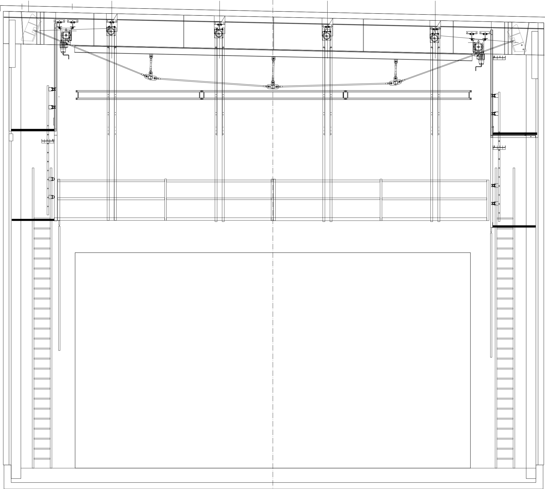
Coupe transversale 1:50 - A3
